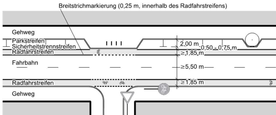
Bild 10: Radfahrstreifen
