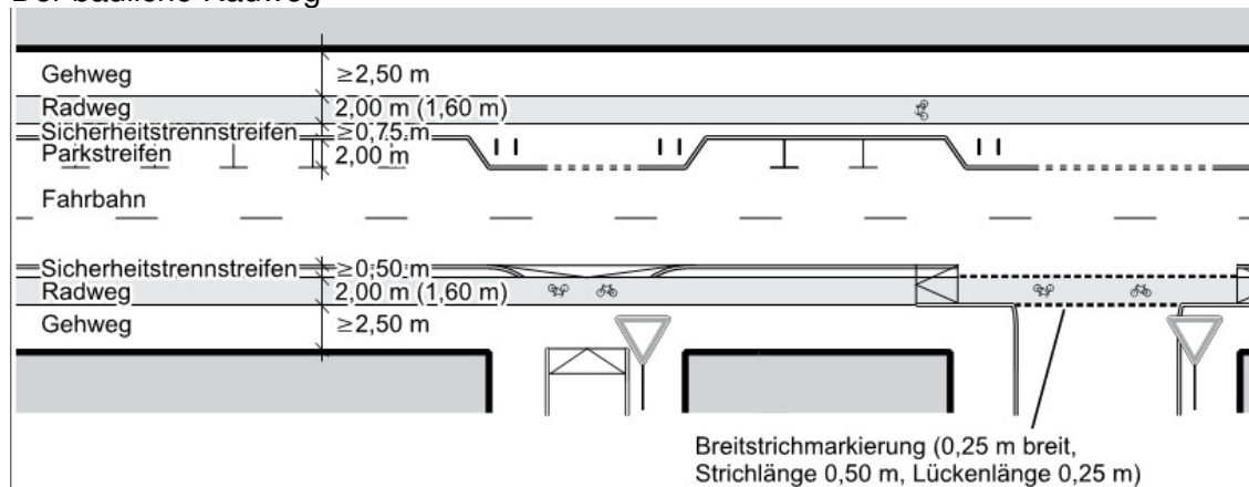
Bild 11: Baulich angelegter Radweg
